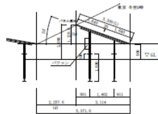
断面図S=1/100
