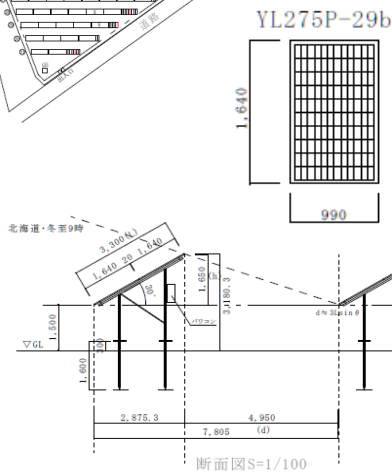
現地詳細図
