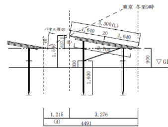
断面図S=1/100
