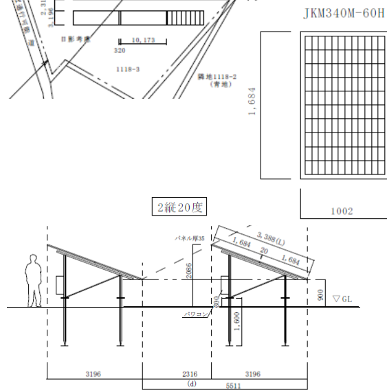
断面図 S=1/100
