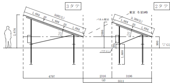
立面図S=1/100
