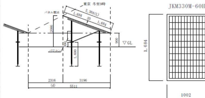
断面図S=1/100
