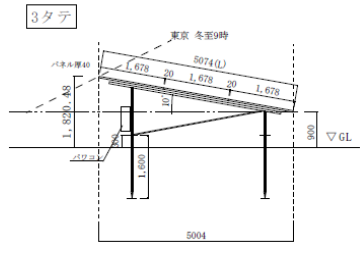
断面図S-1/100
