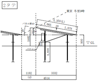
断面図S-1/100
